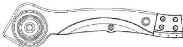
A6P00484 (x1) | GUÍA INFERIOR DERECHA DE 10' VERDE DEL TOBOGÁN
