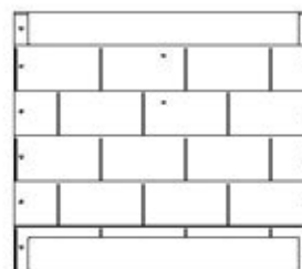
WP6 | PARED CENTRAL IZQUIERDA - W2A03507 (x1) 1 1/4"x18 1/4"x21 1/8" (32x465x536)
